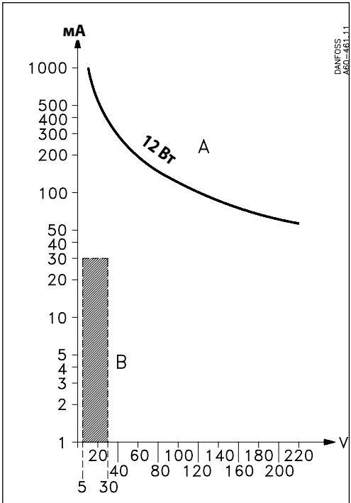
Рис.1 Нагрузка постоянного тока А: максимальная нагрузка Закрашенная область В: приемлемая нагрузка для позолоченных контактов Контактная система: Однополюсный перекидной контакт Материал, контактирующий со средой: Позолоченное серебро Постоянный ток: 12 Вт, 220 В, DC-13 (см. график)
