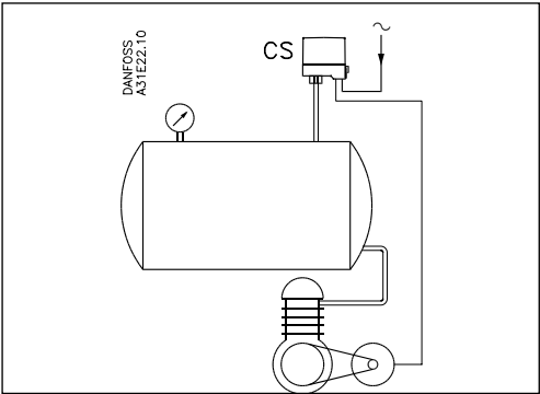
Пример 1 Управление воздушным компрессором с помощью реле CS
