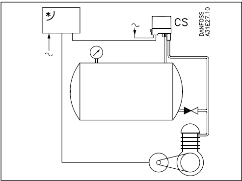
Пример 2 Управление воздушным компрессором с помощью реле CS с установленным перепускным клапаном. Обратите внимание на обратный клапан установленный между перепускной линией и резервуаром
